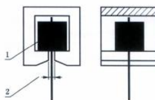
图 A.1 试样尺寸图
