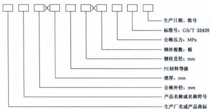
图 4 管材标志图
